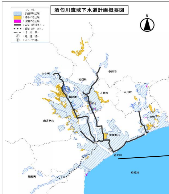
図 2-3 酒匂川流域下水道計画概要図
