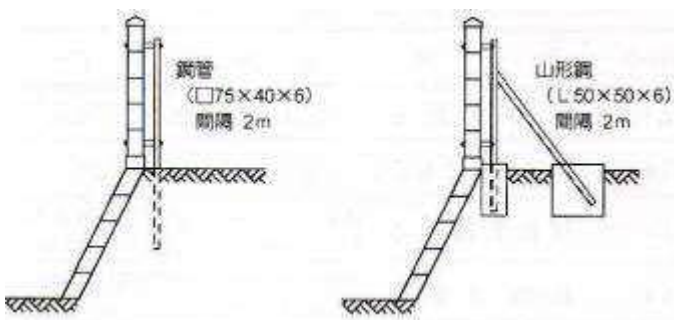
① 鋼柱(鋼管)式
