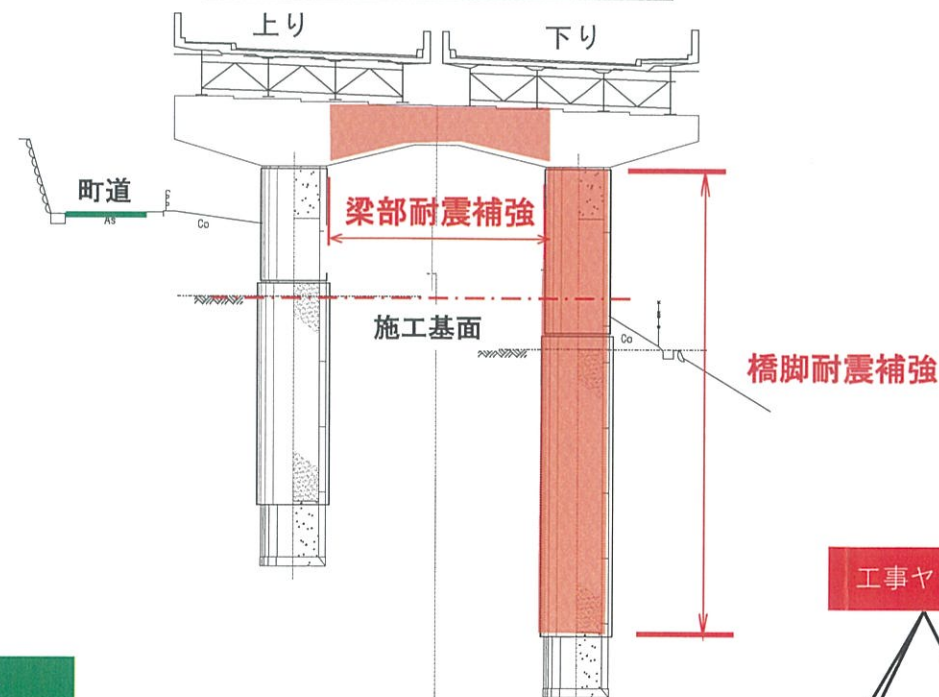
桜ヶ谷陸橋P5橋脚 断面図
