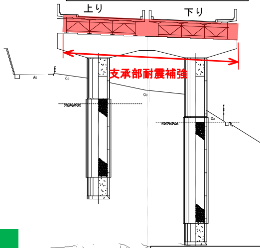
桜ヶ谷陸橋P2, 3橋脚 断面図
